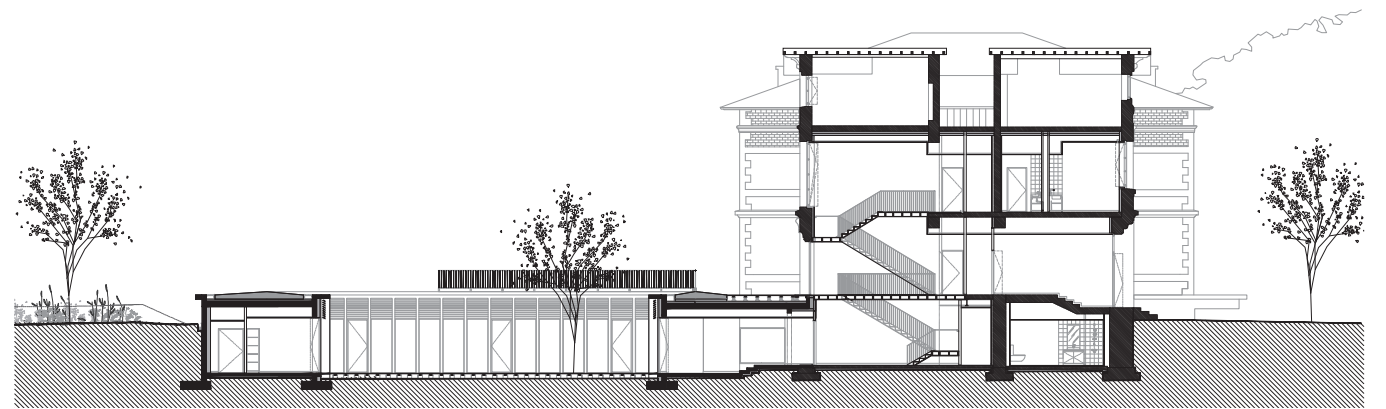
COUPE LONGITUDINALE B
